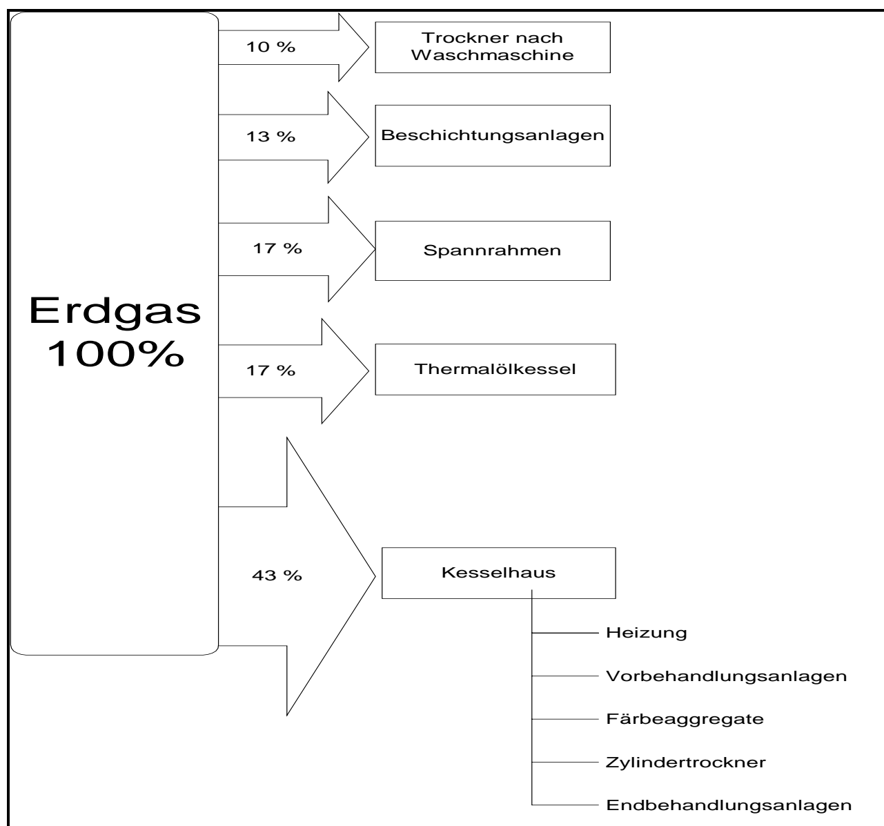
Abbildung 12 – Aufteilung des Gasverbrauchs – Kufner HB 1999
