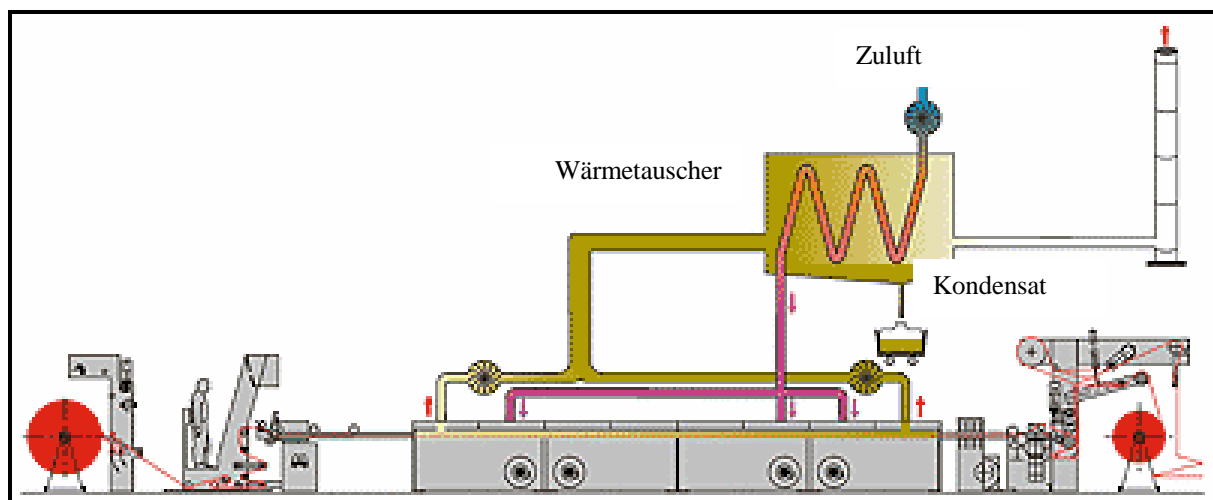
Abbildung 48 – Wärmerückgewinnung mit Trockenluft (Luft/Luft)
