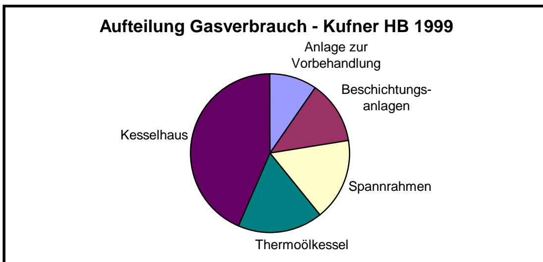
Abbildung 11 - Aufteilung Gasverbrauch - Kufner HB 1999
