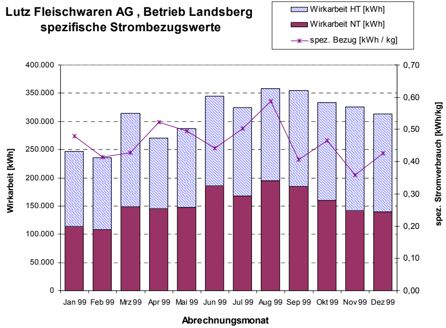
Abbildung 3-3 : spezifischer, auf Produktionsmenge bezogener Strombezug
