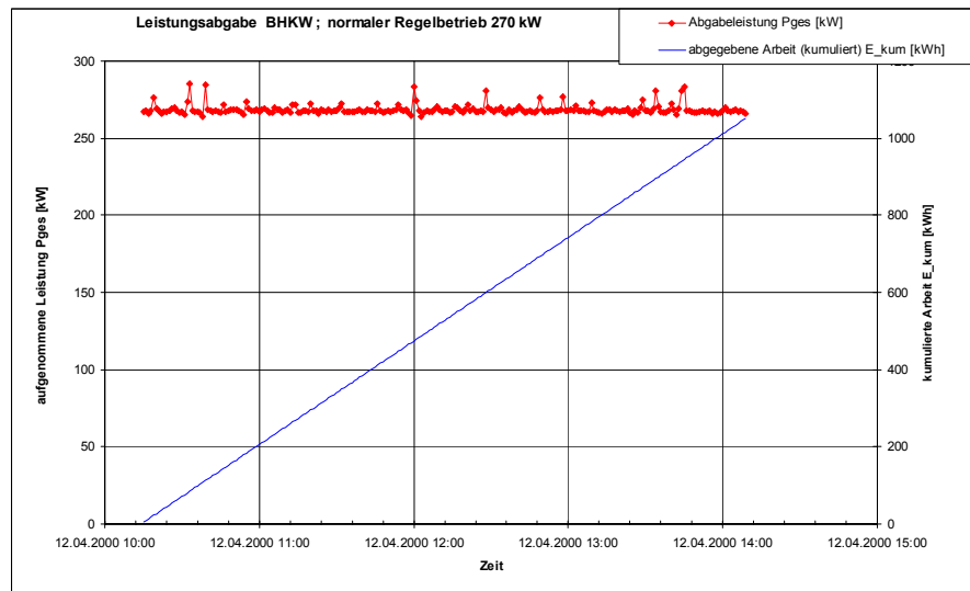
Abbildung 4-1: Leistungsabgabe des BHKW im normalen Regelbetrieb
