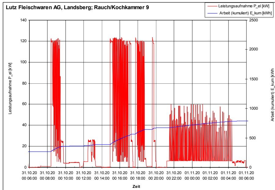
Abbildung 4-7 : Tageslastgang einer Rauch- / Kochkammer mit sechs unterschiedlichen Produktionszyklen
