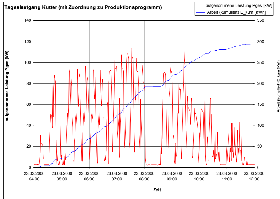
Abbildung 4-6 : Tageslastgang des Kutters. Gleichartige Lastspitzen bei gleichen Produktchargen
