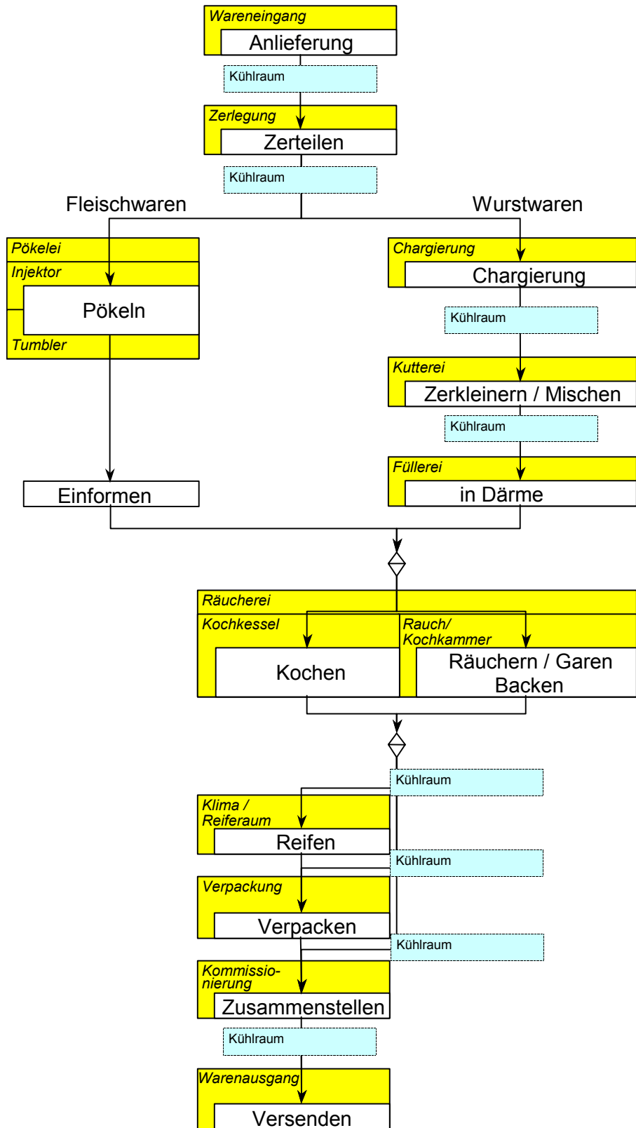
Abbildung 3-1: Produktionsablauf
