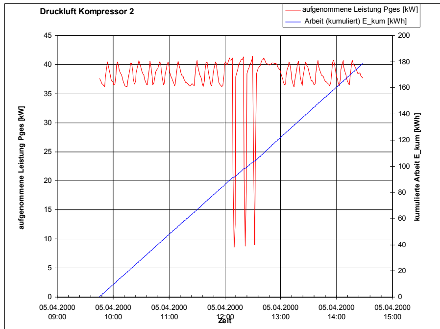
Abbildung 4-3 : Elektrischer Lastgang des Druckluftkompressors 2.
