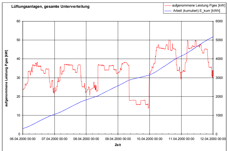
Abbildung 4-4 : Wochenlastgang der Lüftungsanlagen (gesamte Unterverteilung, alle Anlagen)
