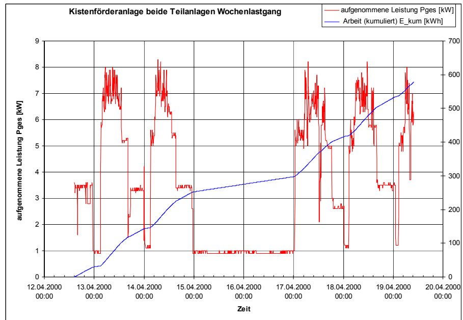
Abbildung 4-5 : Wochenlastgang der Kistenförderanlage
