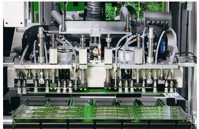
Abb. 8: Platinenproduktion
