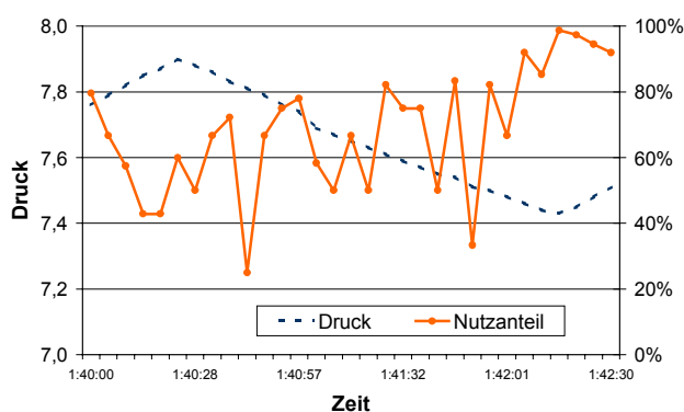
Abb. 8: Leckagemessverfahren bei laufendem Betrieb
