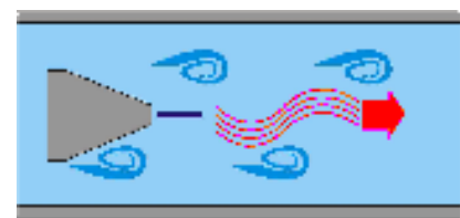
Abb. 5: Karmansche Wirbelstraße
