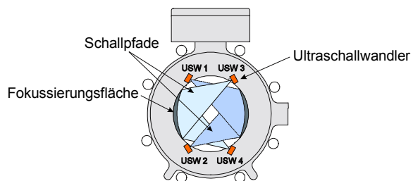
Abb. 6: Ultraschalldurchflussmessung
