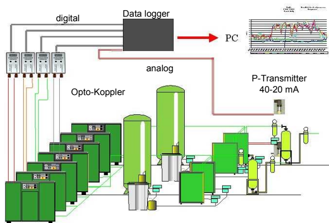
Abb. 7: Digitale Lastzeiterfassung
