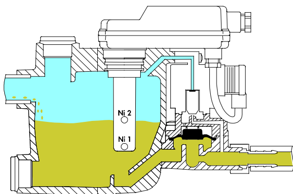
Abb. 10: Niveaugeregelter Ableiter
