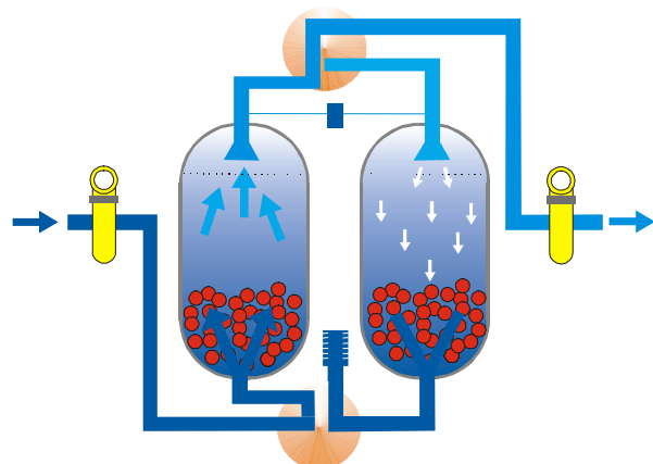
Abb. 4: Kaltregeneration
