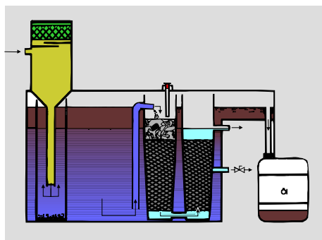
Abb. 11: Statisches Öl-Wasser-Trennsystem
