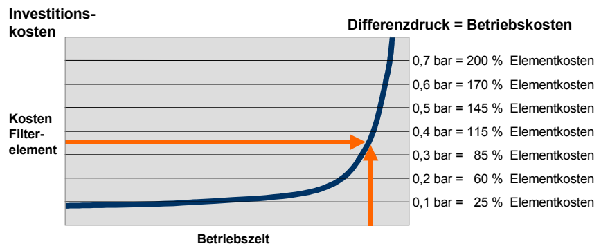
Abb. 7: Typischer Differenzdruckverlauf; Energiekosten in Verhältnis zu Filterelementkosten
