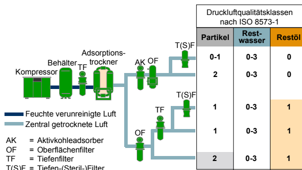
Abb. 13: Druckluftqualitäten bei Einsatz von Adsorptionstrocknern
