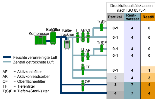
Abb. 12: Druckluftqualitäten bei Einsatz von Kältetrocknern
