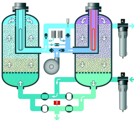
Abb. 5: Warmregeneration
