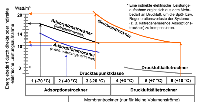
Abb. 1: Verfahren der Lufttrocknung
